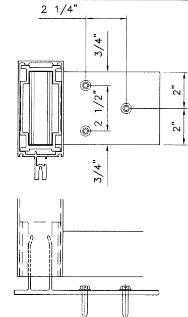
ANCHORS TYPE 'C' JAMB ANCHORS ('F' CLIP ES-7525-51)
