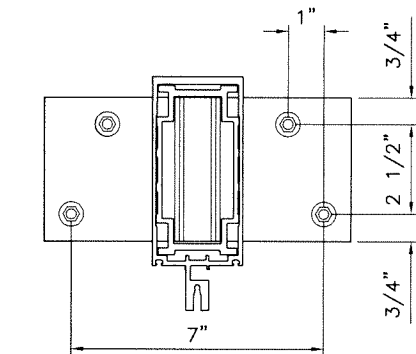
ANCHORS TYPE 'A' JAMB ANCHORS ('F' CLIP ES-7525-51)
