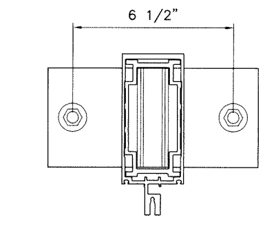
ANCHORS TYPE 'B' JAMB ANCHORS ('F' CLIP ES-7525-51)
